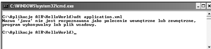
Rysunek 2.22. Jeśli aplikacja adl nie może znaleźć Java Runtime Environment (JRE), prawdopodobnie zobaczysz taką informację o błędzie
